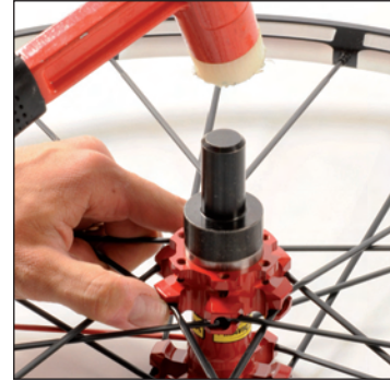
Neue Lager mithilfe der Lager-Montagewerkzeuge 323 945 01 (rechts) und M40218 (links) einbauen.
