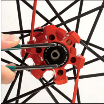
Lager-Abdeckkappe mithilfe des Stiftschlüssels losdrehen.
