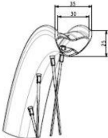
Jante arrière E-Crosstrail Carbone SL
