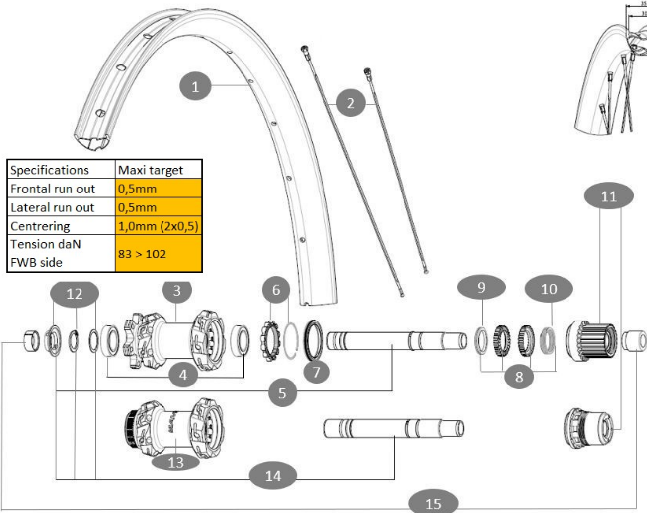
Jante arrière E-Crosstrail Carbone SL
