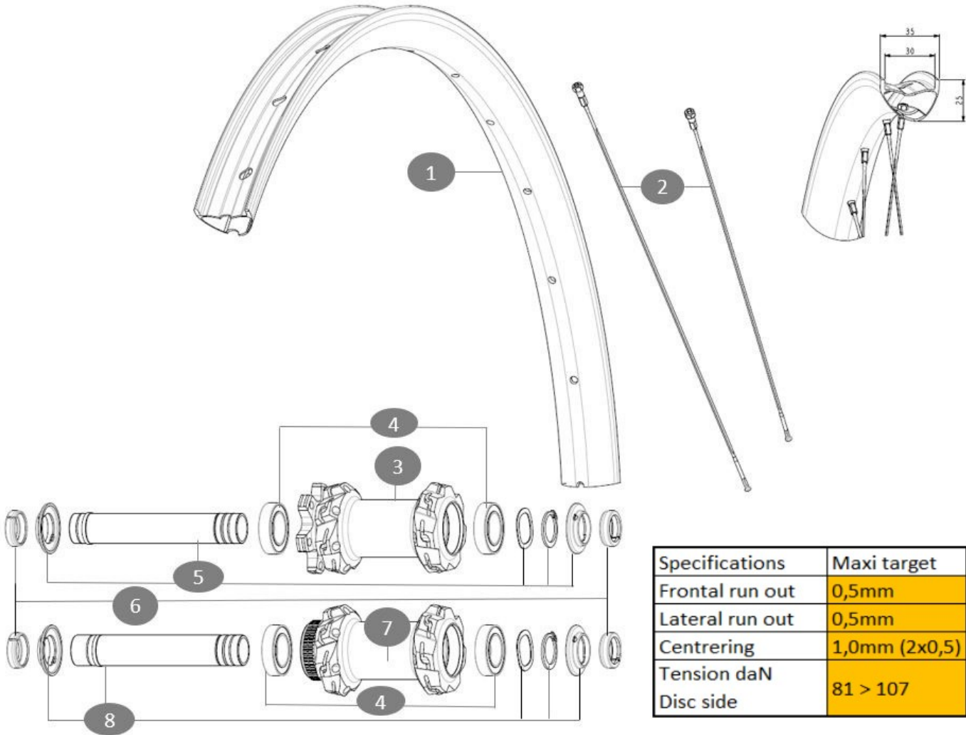
Jante avant E-Crosstrail Carbone SL
